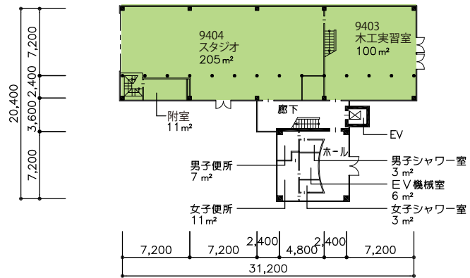
1階
