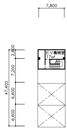
塔屋
