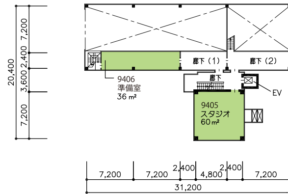
2階
