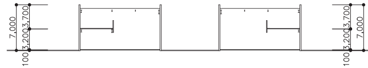
B-B 断面
