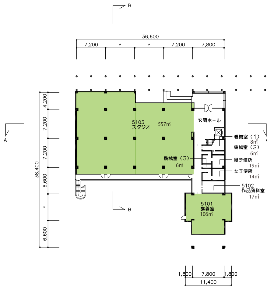
1 階
