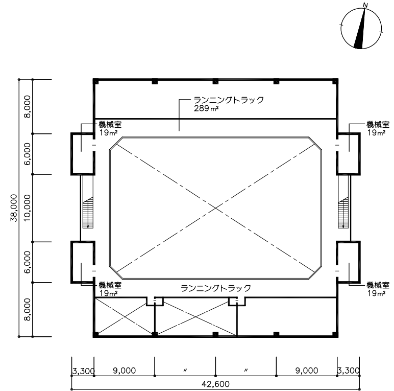
2階
